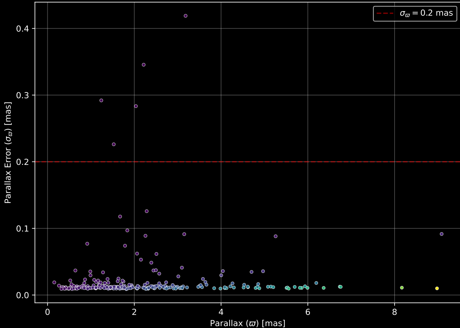
GALAH DR4 Field: [7129] Parallax Quality (n= 262)
