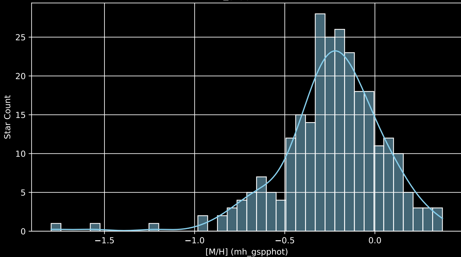
GALAH DR4 Field: [7129] [M/H] (mh_gspphot) (n= 261)
