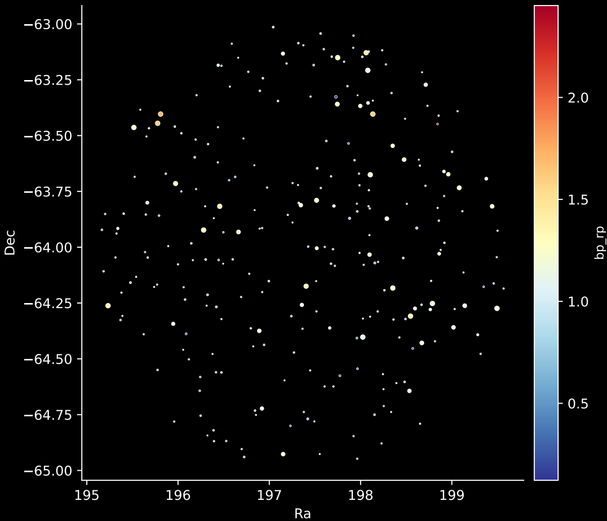
GALAH DR4 Field: [7129] Stars: 262
